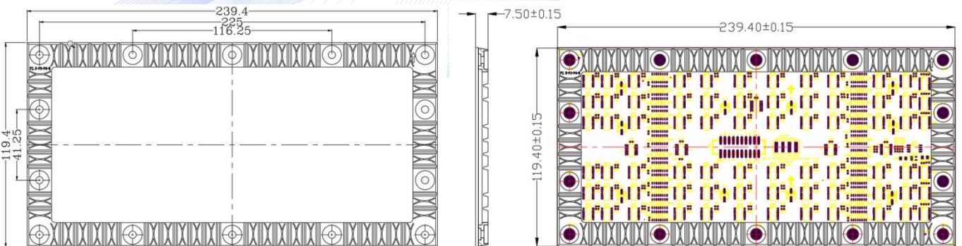
模组孔位图 (软底壳磁铁分排图)
